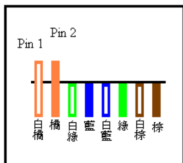
RJ45
